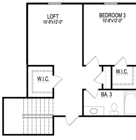
Optional Bedroom 3
